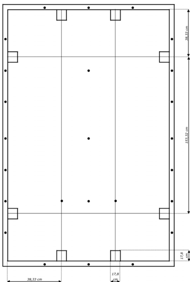
Tekening 6 afmetingen ankerkader 38/2
