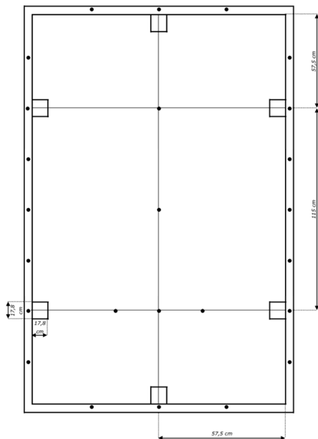
Tekening 7 afmetingen ankerkader 57/2
